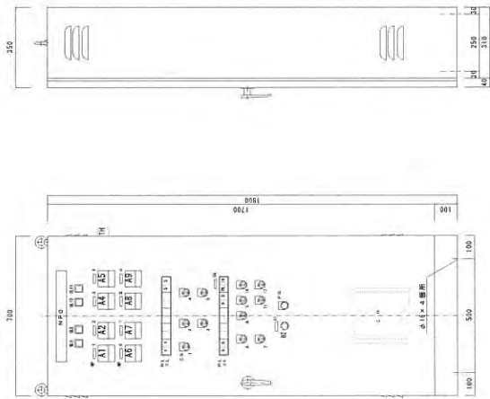
制御盤外形図 1/1.0
